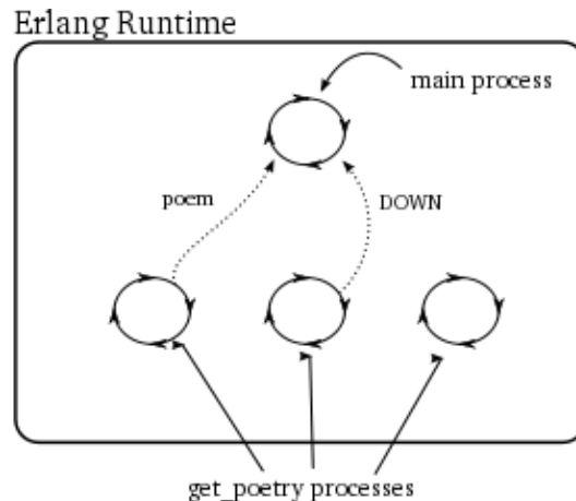
Рис. 45: Поэтический клиент на Erlang
